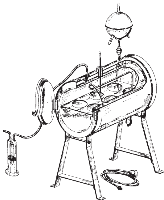
FIG. 1 Moisture Oven
